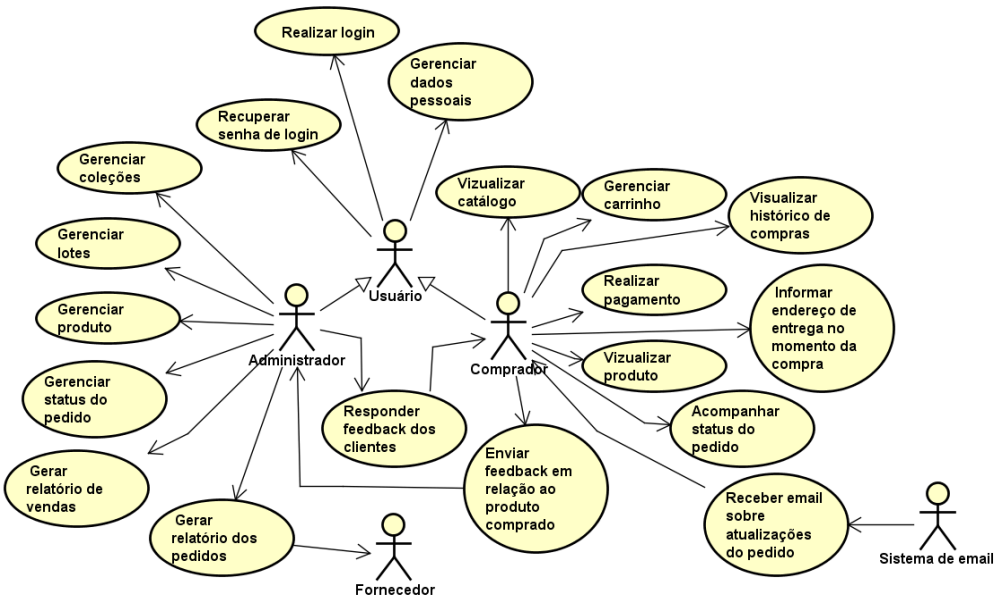
Imagem 5 - Diagrama de casos de uso
