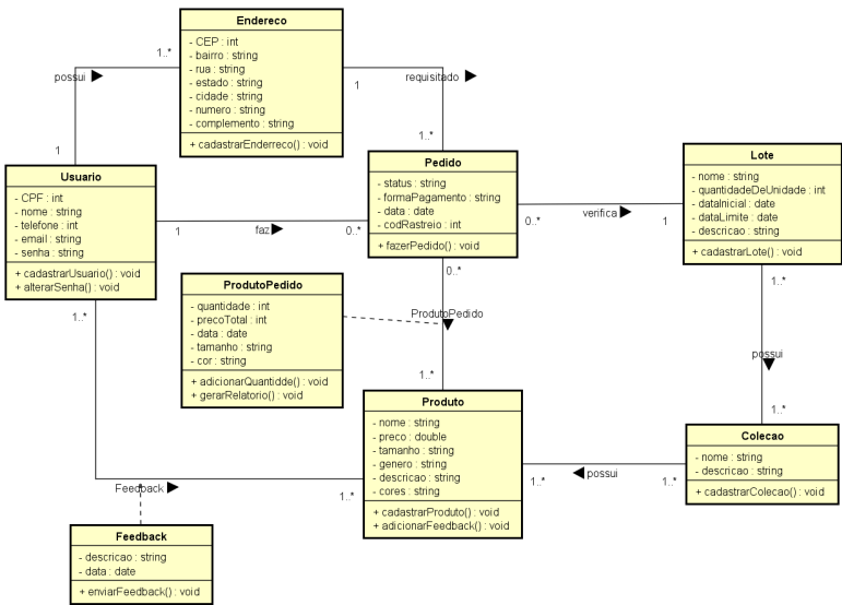
Imagem 4 - Diagrama de classes
